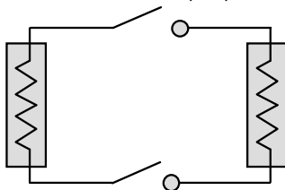
B: Verkabelung Wasserpumpe der Wärmepumpe
