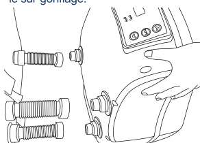
8) Raccordez le bloc moteur au bassin à l'aide des trois raccords à visser.
