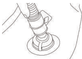
4) Raccordez l'autre extrémité du tuyau à la valve d'air située sur le bassin
