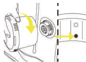
10) Mets le filtre du cartouche dans un support avant de le visser sur l'appareil pour succion dans l'évier.
