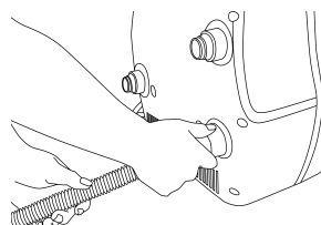
3) Raccordez une extrémité du tuyau de gonflage au bloc moteur sur la sortie.
