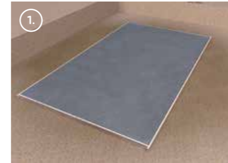
1. Betonplateau 15 cm gieten met wapeningsnet 8/8/150/150
